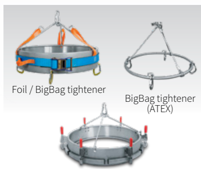
Foil tightener (ATEX)
