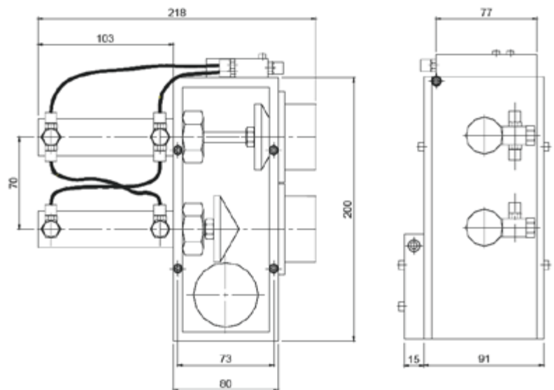
Maßskizze RS 2000
